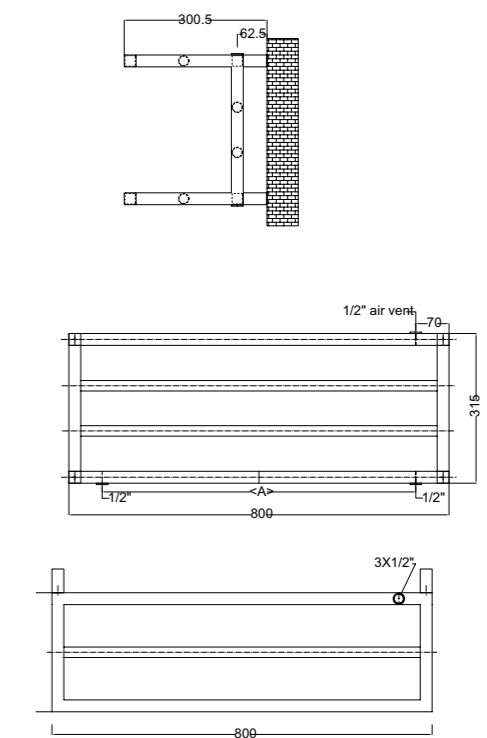
SMART U welded/sudat (for RAL and stainless steel / pentru vopsit și inox)
